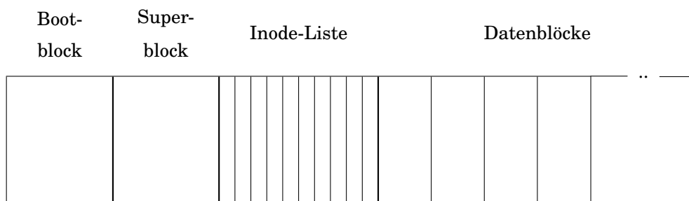
Abb. 2.3: UNIX-Datei-System, Sicht von unten
