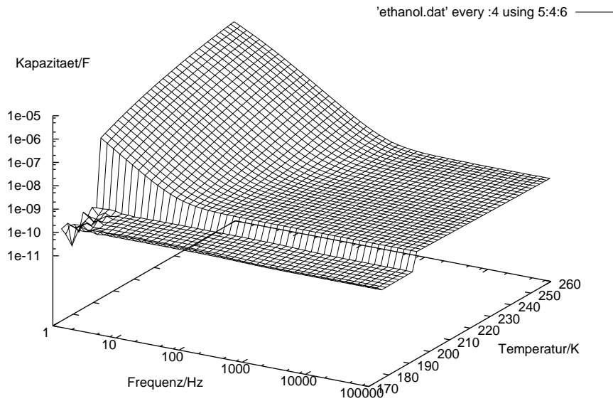
Abb. 2.11: Versuchsdaten, dargestellt mittels gnuplot
